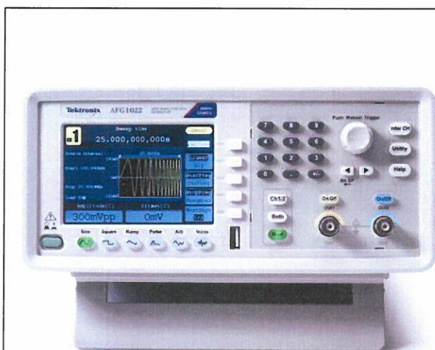
Рисунок 1 – Вид передней панели
